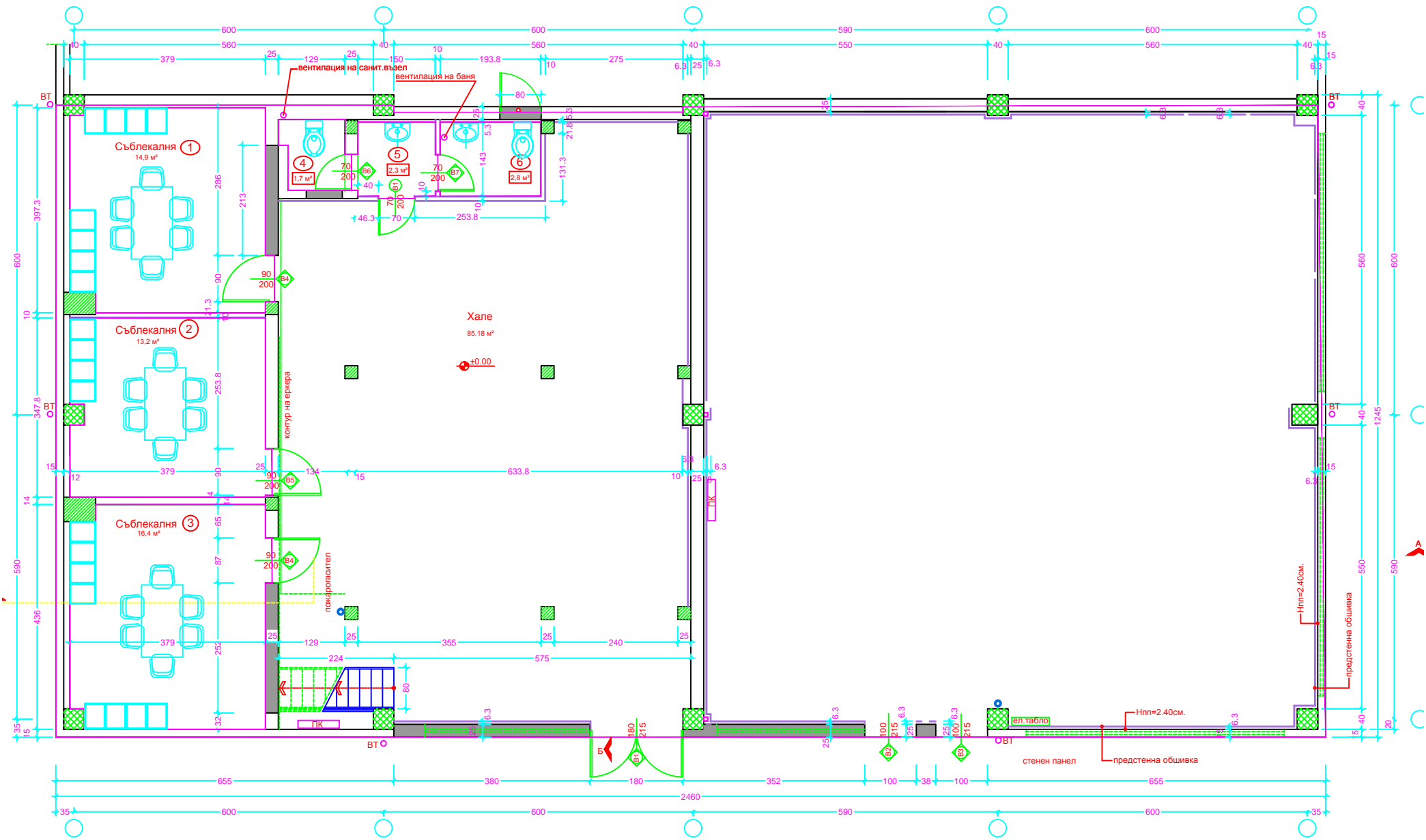
ПЛАН ПЪРВИ ЕТАЖ, КОТА ±0.00 Застроена площ: 300м2
