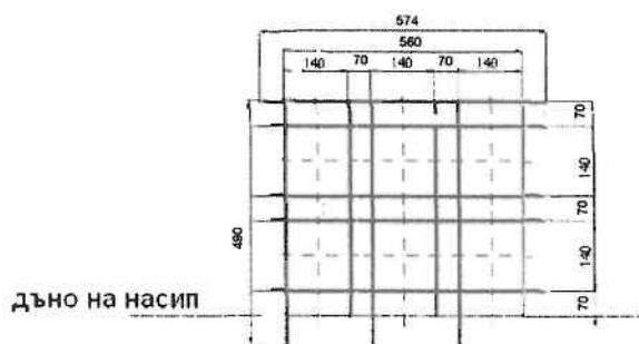
Решетка от арматурна стомана №8
