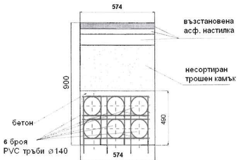
Тръбна мрежа при пресичане на улично платно
