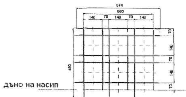
Решетка от арматурна стомана №8
