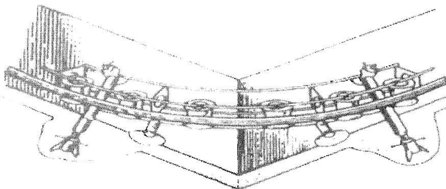
Ъглово ролково устройство за обхождане на ъгъл
