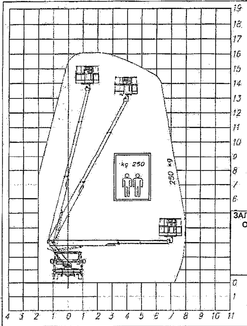
РАБОТНА ДИАГРАМА ТЗ1Б
